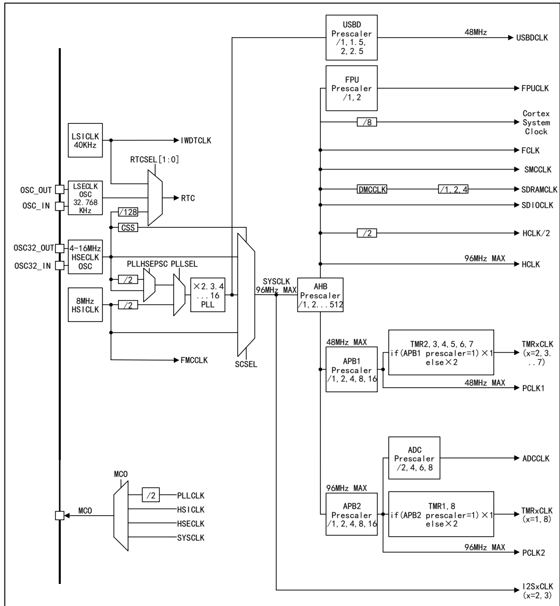
图 6 APM32F103xCxDxE 时钟树
