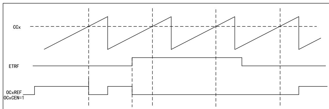
图 43 OCxREF 时序图
