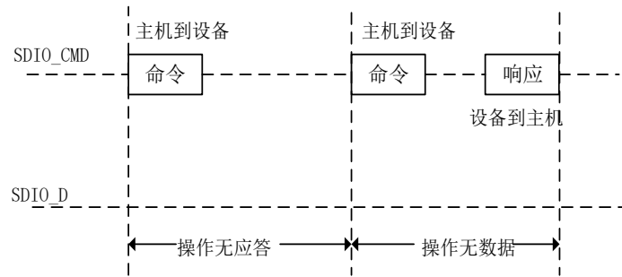
图 120 SDIO (多) 数据块读操作
