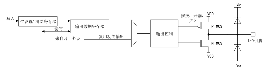
图 21 输出模式 I/O 结构
