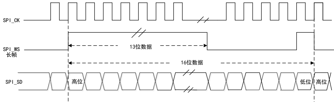
图 107 PCM 标准波形
