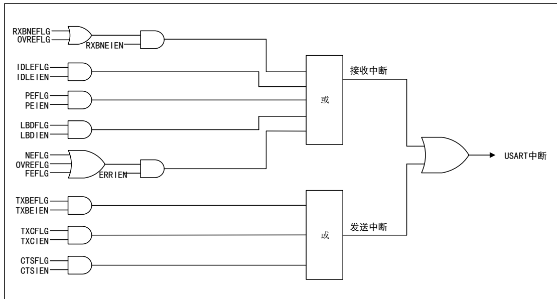
图 76 USART 中断映射
