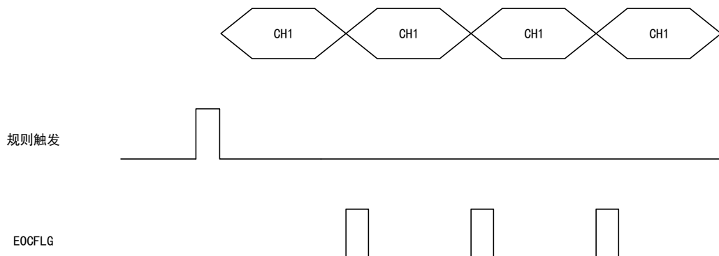
图 127 连续转换模式时序图
