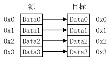
图 10 源为 8bits 目标为 8bits 的传输宽度
