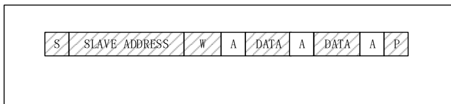
图 79 主机写数据到从机
