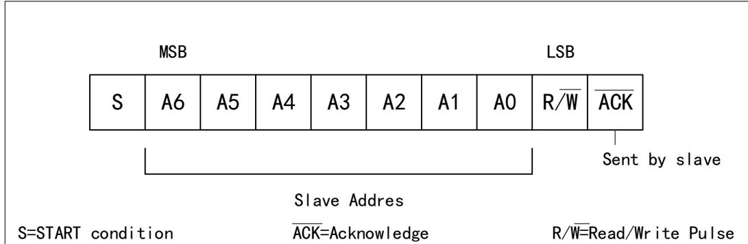
图 86 7 位地址格式
