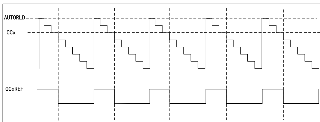
图 52 PWM2 向下计数模式的时序图
