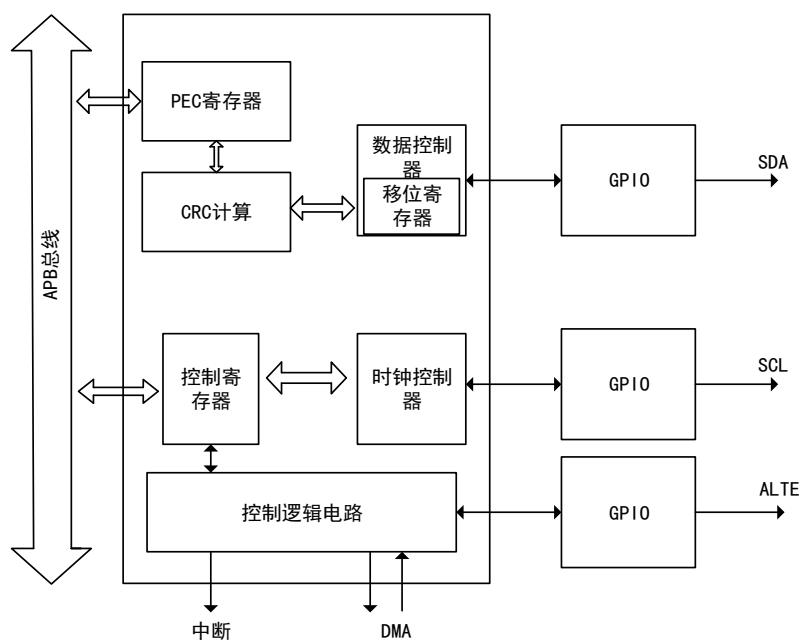
图 77 I2C 功能结构图
