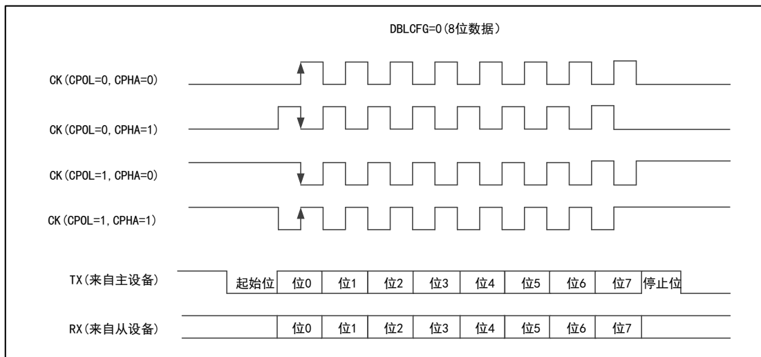
图 69 USART 同步传输时序图 (DBLCFG=0)
