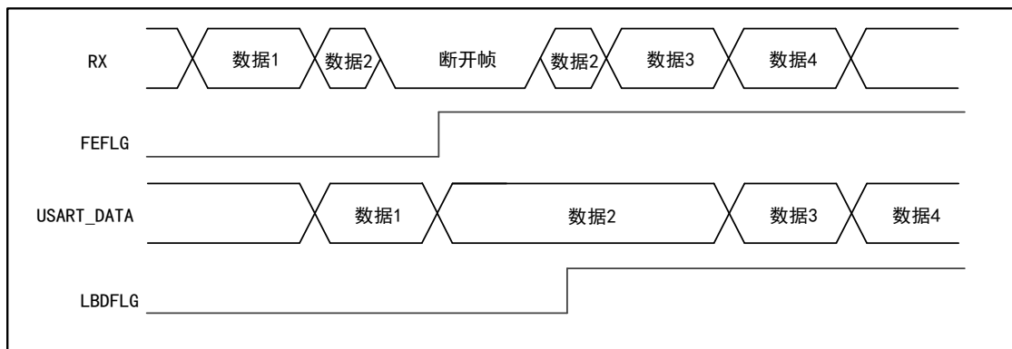
图 72 数据传输状态检测断开帧
