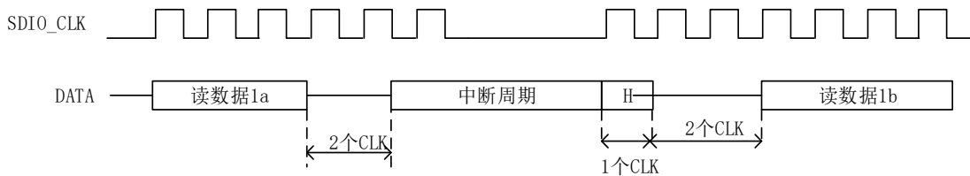
图 125 通过停止 SDIO_CLK 的读等待操作
