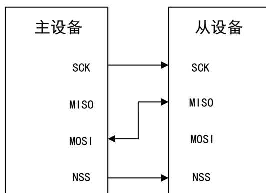
图 97 双向线连接
