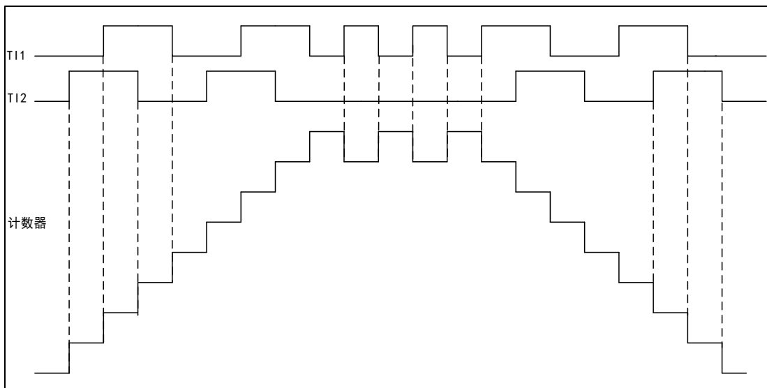
图 56 编码器模式下的计数器操作实例
