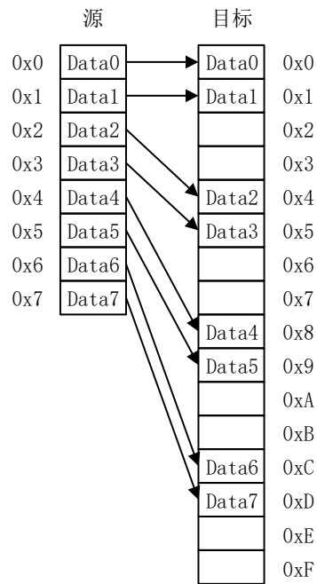
图 15 源为 16bits 目标为 32bits 的传输宽度
