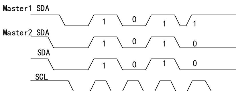
图 84 SDA 时序图
