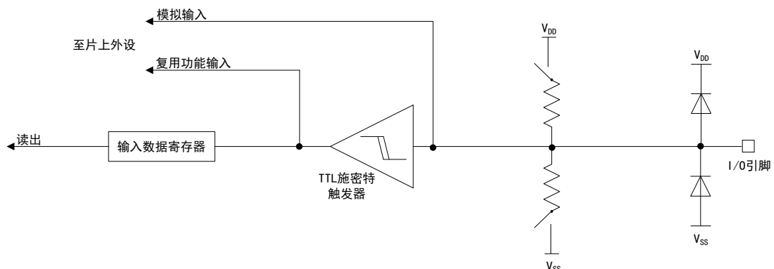
图 20 输入模式结构
