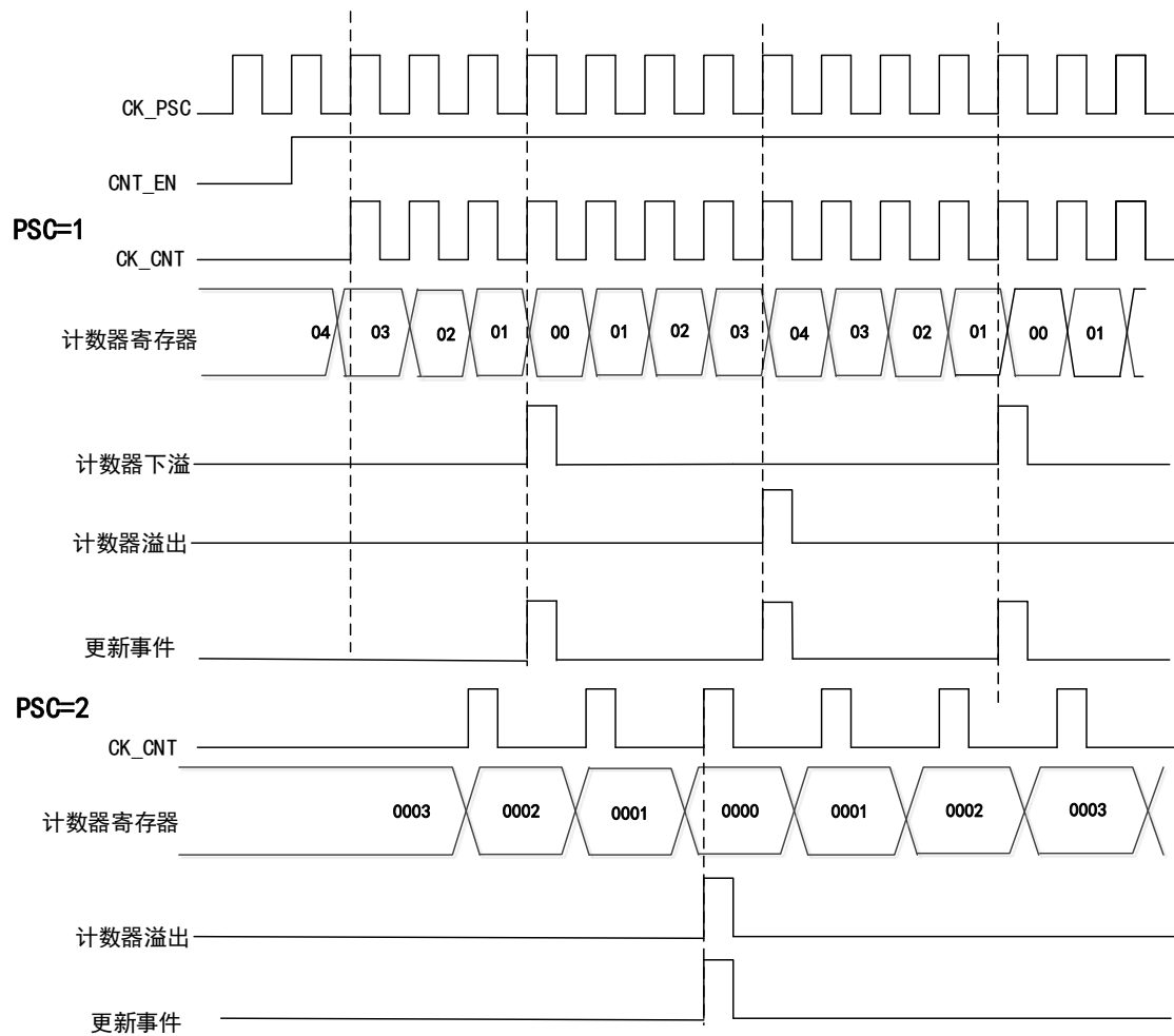
图 26 中央对齐模式下，分频因子为 1 或 2 的时序图
