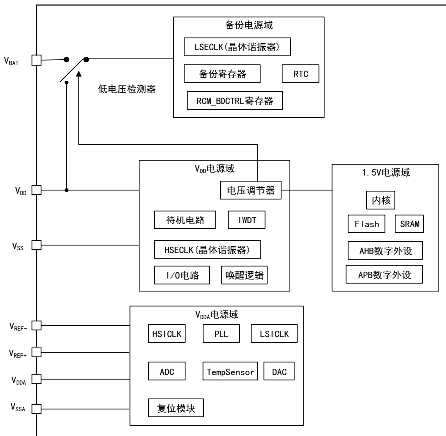
图 7 电源控制结构框图
