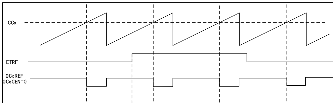
图 42 OCxREF 时序图
